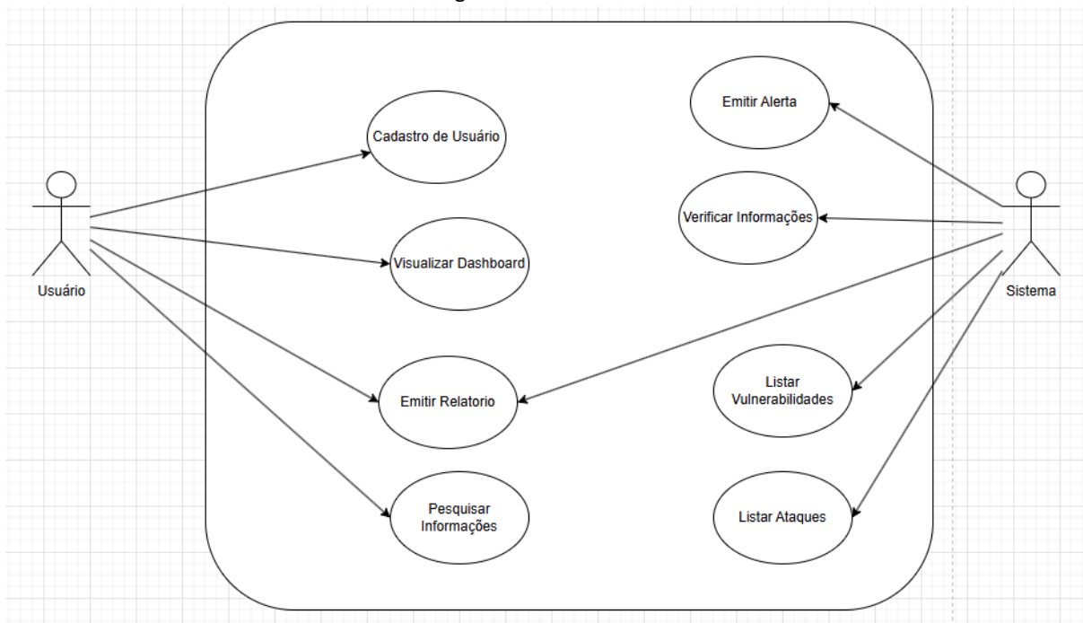
Figura 2 - Caso de Uso
